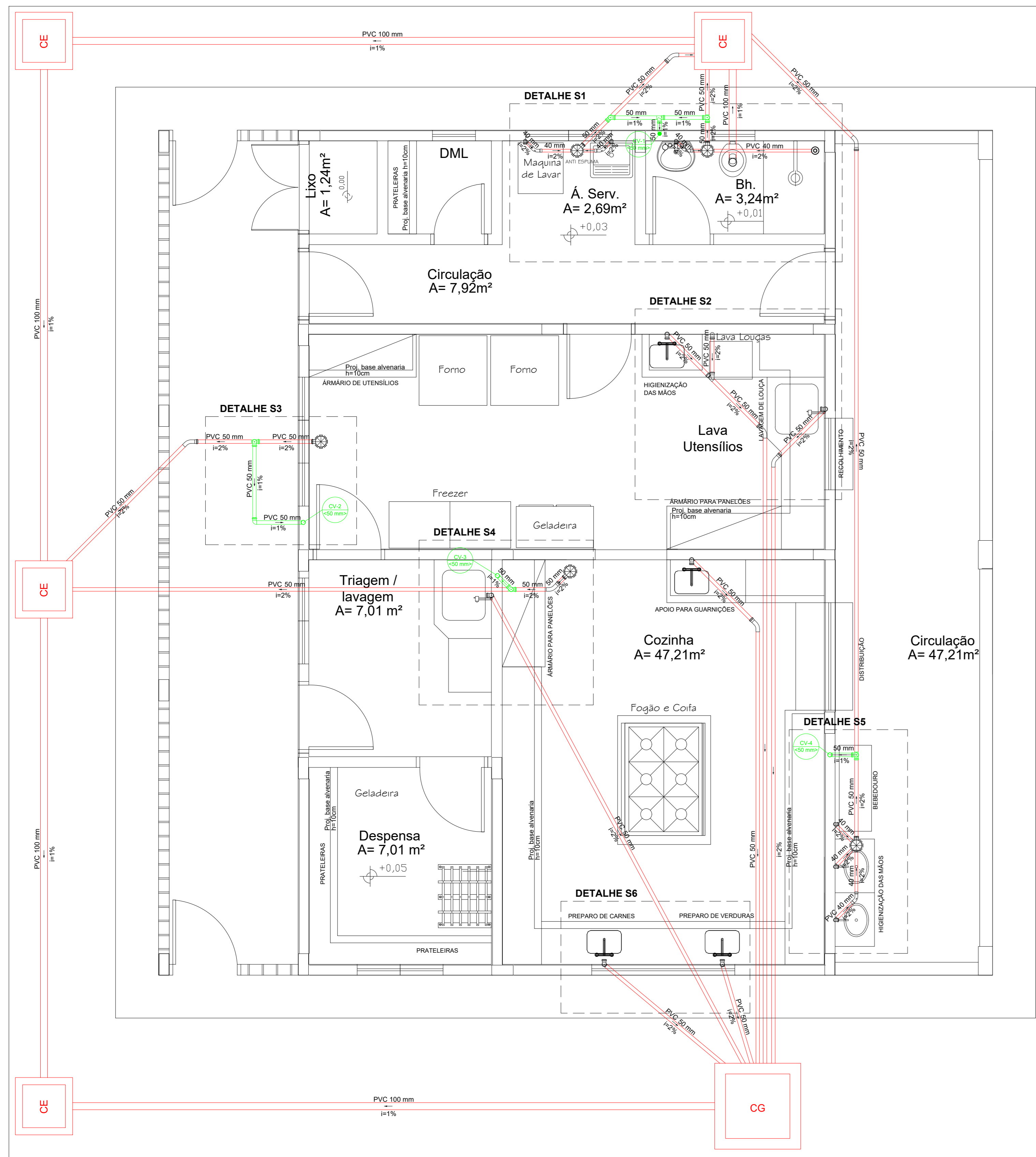
Planta do Terreo - Esgoto Escala 1:50
